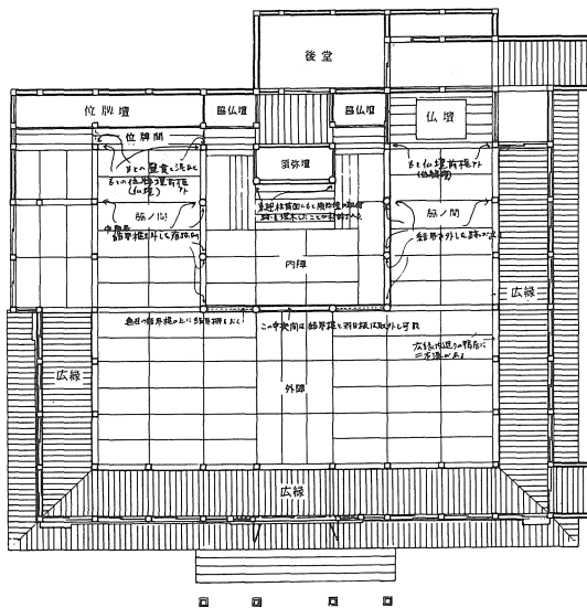
図1 観音寺本堂現状図
