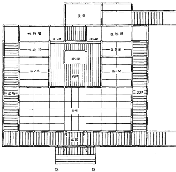
図2 観音寺本堂復原図
