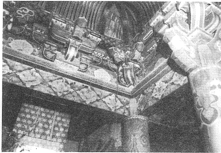
写真12 内陣左脇仏壇前出組斗拱
