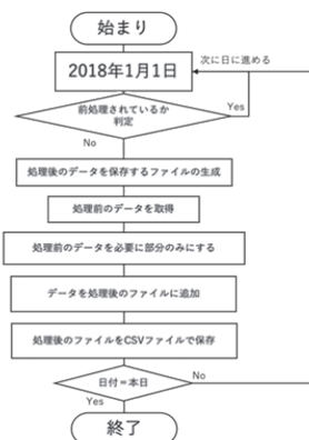
図1. データ処理プログラムのフローチャート
