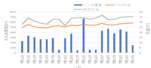
図5 夏季における1号館のガス消費量変化
