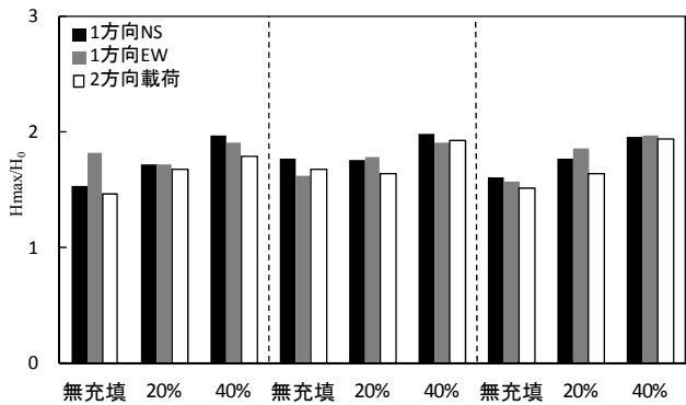
図-12 最大荷重の比較
