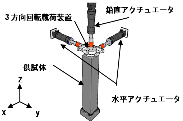
図-2 3次元載荷システム
