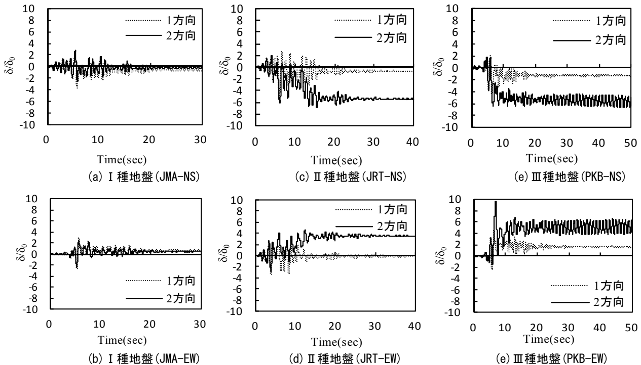
図-6 1方向および2方向載荷時の応答変位時刻歴(20%充填)
