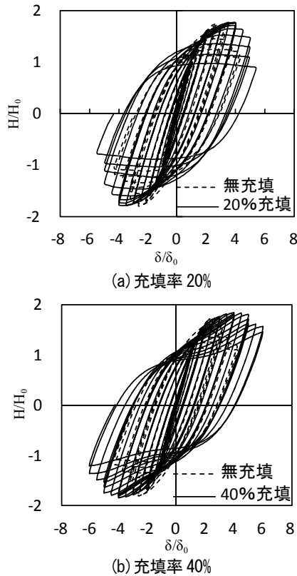
図-3 水平荷重-変位曲線
