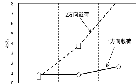
(Ⅰ種地盤) (Ⅱ種地盤) (Ⅲ種地盤) 図-11 残留変位の比較(平均値)
