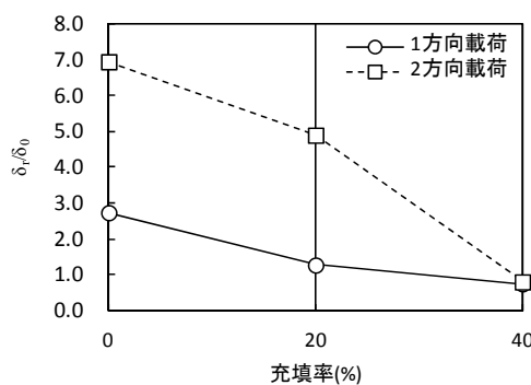
図-16 残留変位の比較
