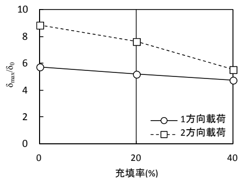
図-15 最大応答変位の比較
