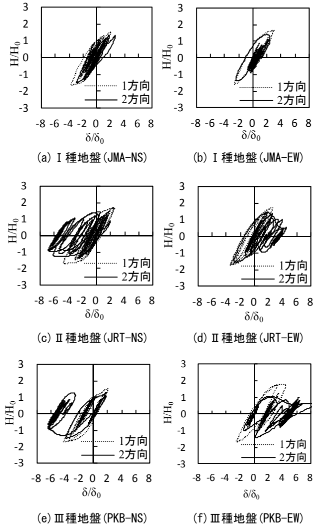
図-5 水平荷重-水平変位履歴曲線(20%充填)
