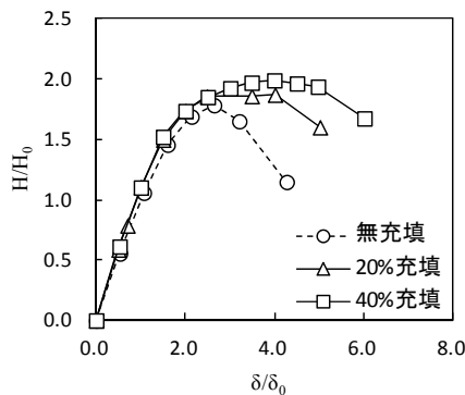
図-4 包絡線
