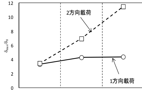
(Ⅰ種地盤) (Ⅱ種地盤) (Ⅲ種地盤) 図-10 最大応答変位の比較(平均値)
