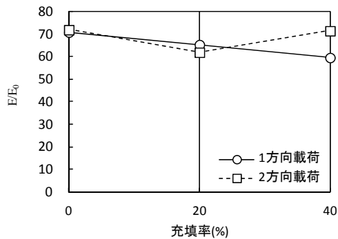
図-18 エネルギー吸収量の比較
