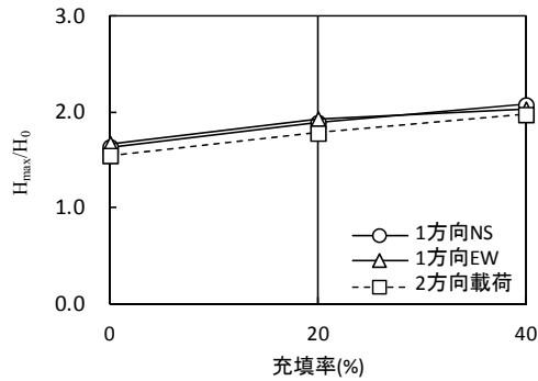
図-17 最大荷重の比較
